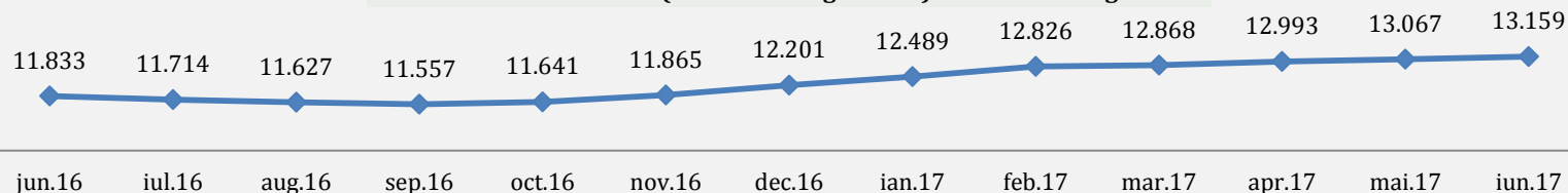
Gaze naturale vehiculate (inclusiv înmagazinare) - mil.mc - rolling 12 luni
