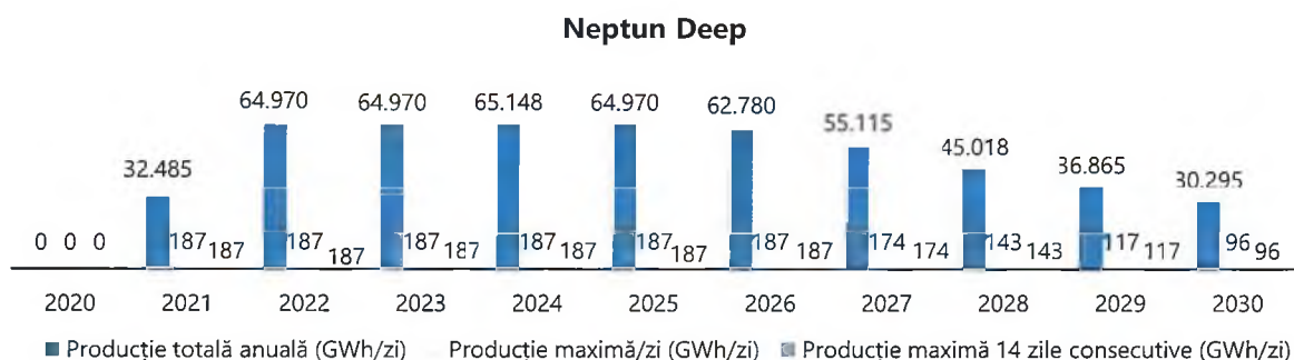
Grafic 18 – Proгноza producției de gaze naturale Exxon Mobil în perioada 2020–2030
