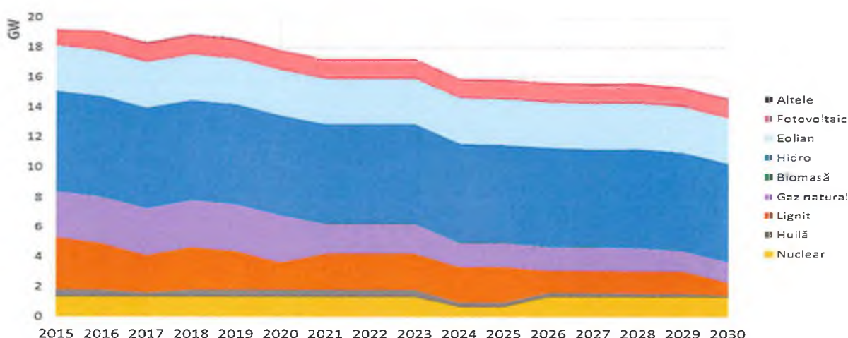
Grafic 7 –Evoluția parcului de capacități producție energie electrică disponibile, fără investiții în capacități noi Sursa: Strategia energetică a României 2019–2030 cu perspectiva anului 2050 - proiect
