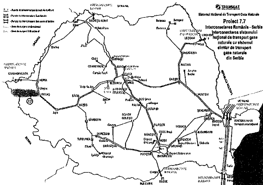
Figura 14 - Interconectarea SNT cu Serbia pe direcția Receaș–Mokrin
