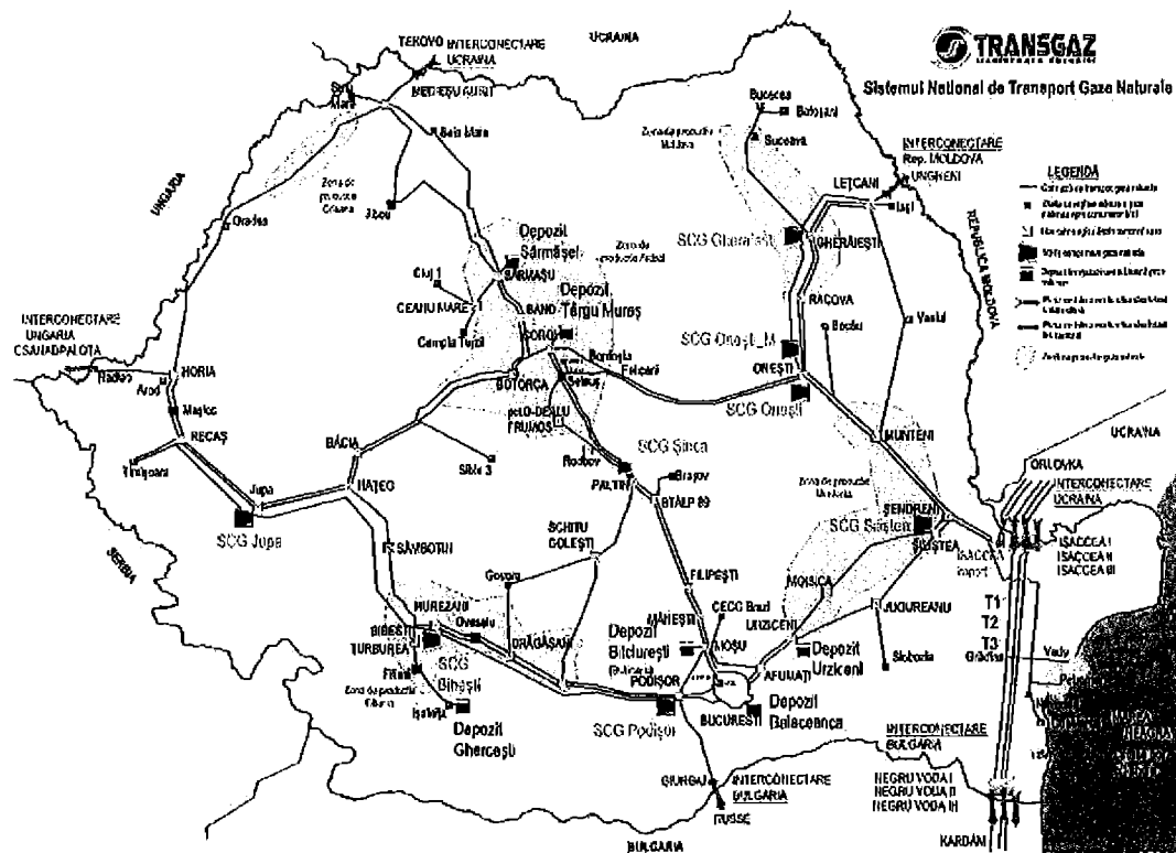
Figura 2 - Harta Sistemului Național de Transport Gaze Naturale
