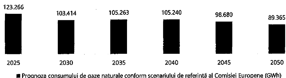
Grafic 9 – Prognoza consumului de gaze naturale în perioada 2025 -2050 conform Scenariului de referință al Comisiei Europene (GWh/an)
