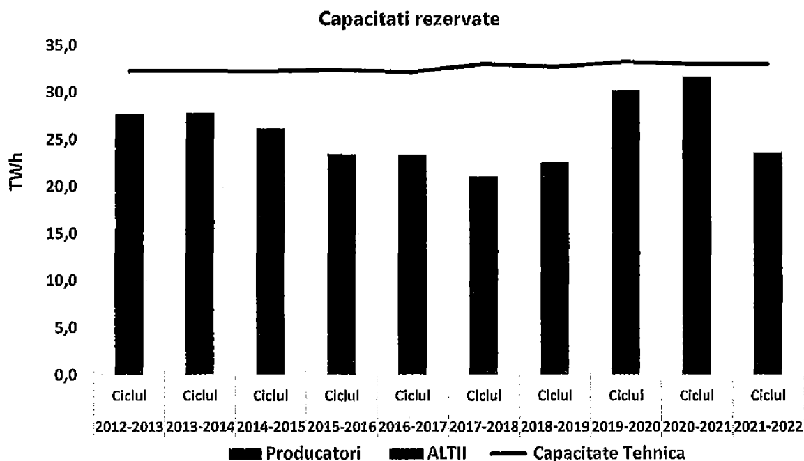
Grafic 18- Capacitățile rezervate în perioada 2012-2022
