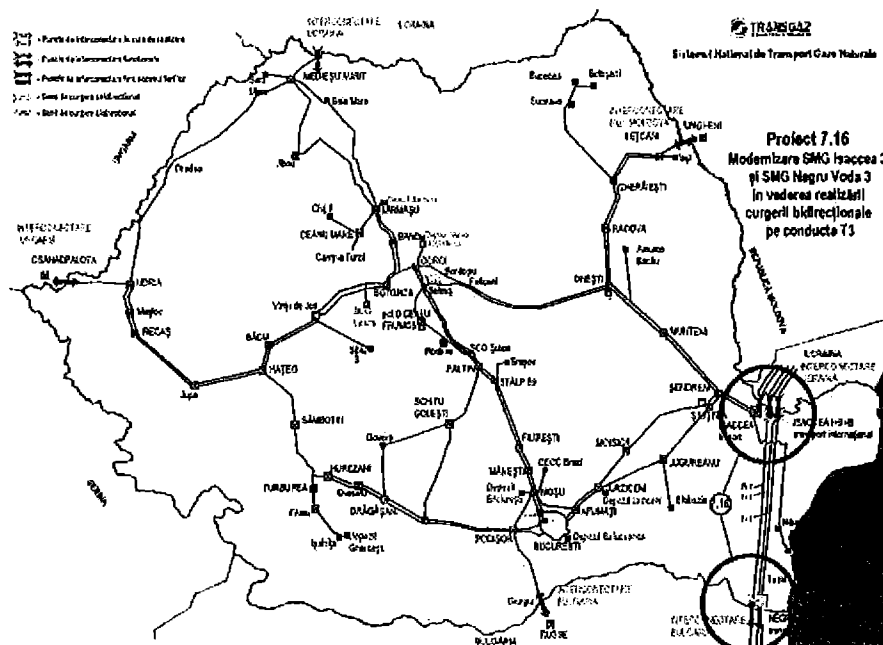
Figura 19- Modernizare SMG Isaccea 3 și SMG Negru Voda 3 în vederea realizării curgerii bidirecționale pe conducta T3
