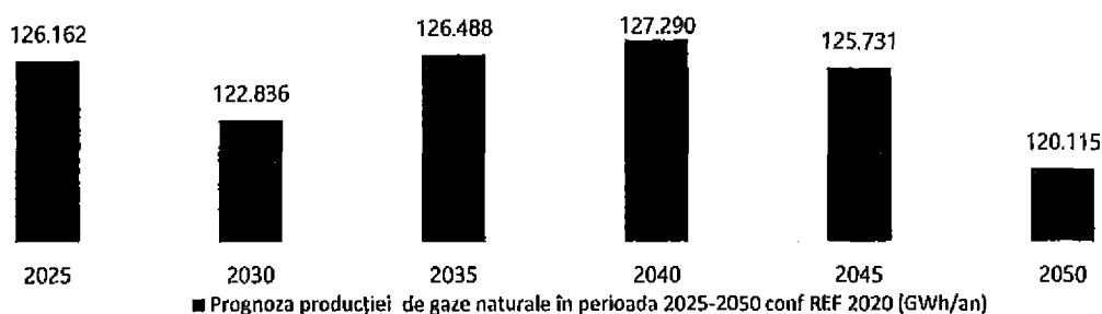
Grafic 12 – Prognosticele de gaze naturale în perioada 2025-2050 conform Scenariului de referință al Comisiei Europene (REF 2020)
