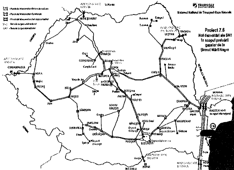
Figura 13 - Dezvoltări ale SNT în Marea Neagră
