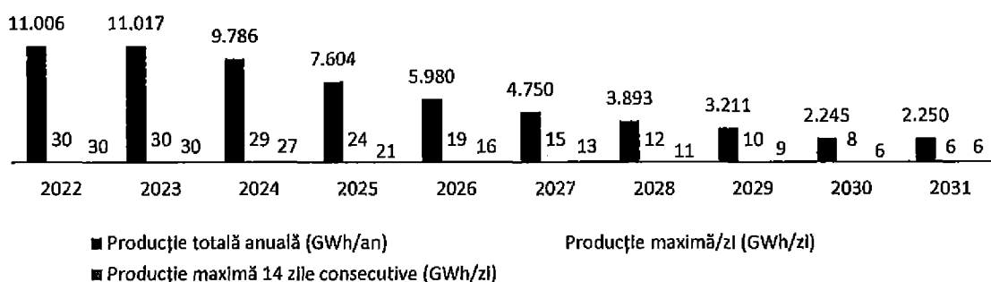
Grafic 14– Prognoza producției de gaze naturale Black Sea Oil and Gas în perioada 2022–2031
