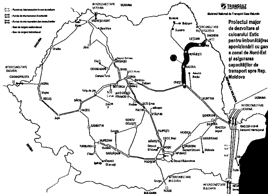
Figura 13 - Dezvoltări ale SNT în zona de Nord-Est a României
