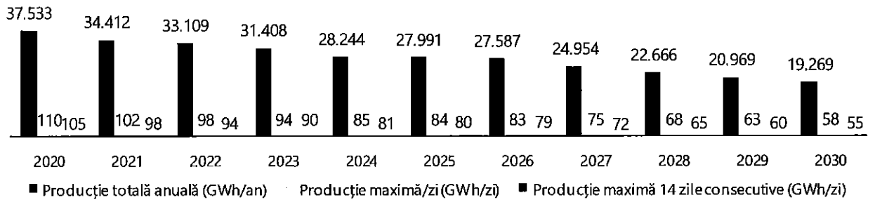
Grafic 16– Prognoza producției de gaze naturale OMV Petrom în perioada 2020–2030
