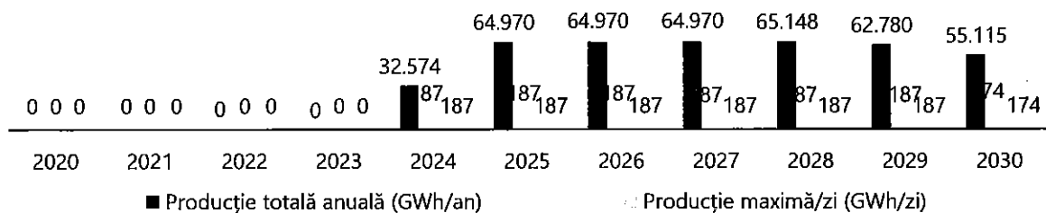
Grafic 17 – Prognoza producției de gaze naturale Exxon Mobil în perioada 2020–2030
