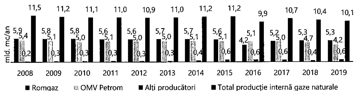
Grafic 11 – Producția internă de gaze naturale în funcție de principalii producători în perioada 2008-2019 (mld mc/an) Sursa: Intern - Dispererat
