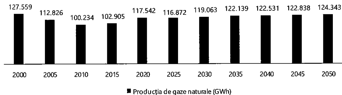
Grafic 13 – Prognoza producției de gaze naturale în perioada 2000–2050 conform Scenariului de referință al Comisiei Europene
