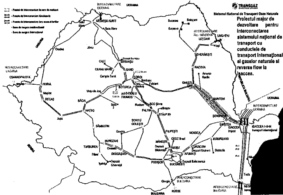
Figura 12 - Harta proiectului major de dezvoltare pentru interconectarea SNT cu conducta de transport internațional Transit 1 și reverse flow Isaccea
