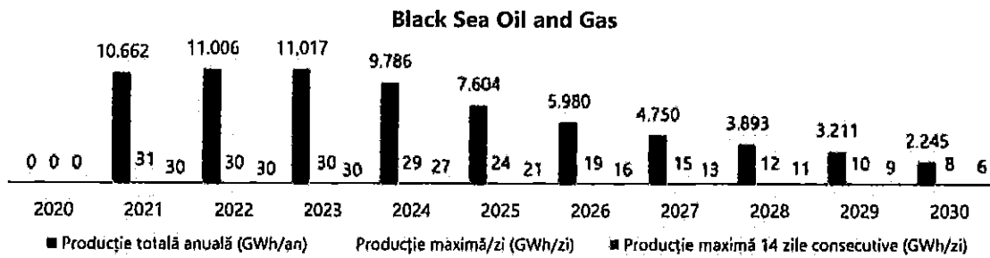
Grafic 16– Proгноza producției de gaze naturale Black Sea Oil and Gas în perioada 2020–2030
