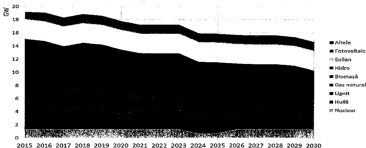
Grafic 7–Evoluția parcului de capacități producție energie electrică disponibile, fără investiții în capacități noi Sursa: Strategia energetică a României 2019–2030 cu perspectiva anului 2050
