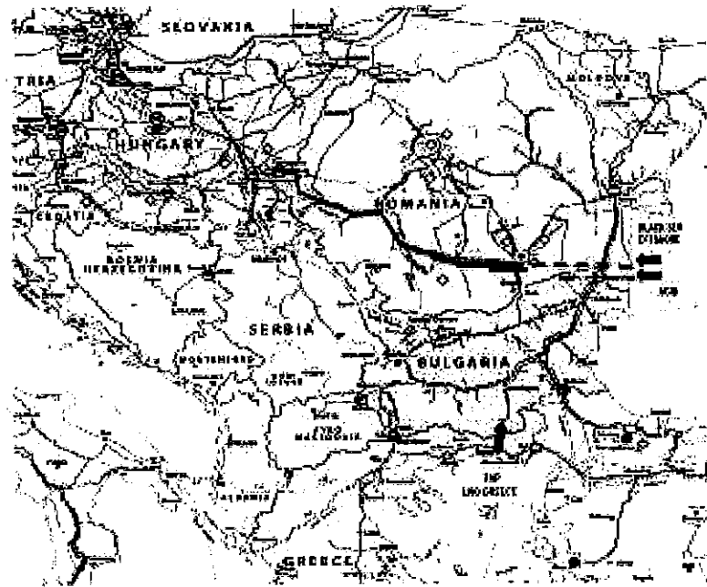
Figura 1 - Punctele de interconectare ale sistemului românesc de transport gaze naturale cu sistemele similare ale Bulgariei și Ungariei
