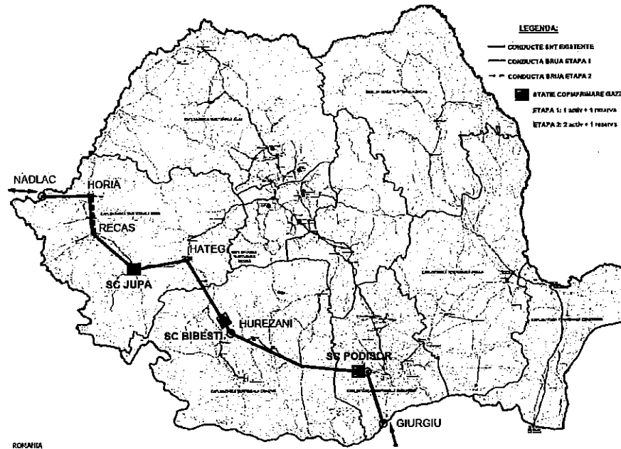
Figura 3 – Harta proiectului major de dezvoltare al coridorului Bulgaria-România-Ungaria-Austria – Faza II
